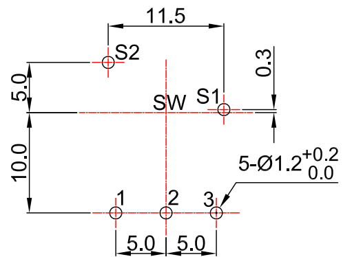
安装孔位置图 P.C.B. mounting hole detail
