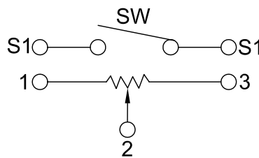
接线图 Circuit explanation
