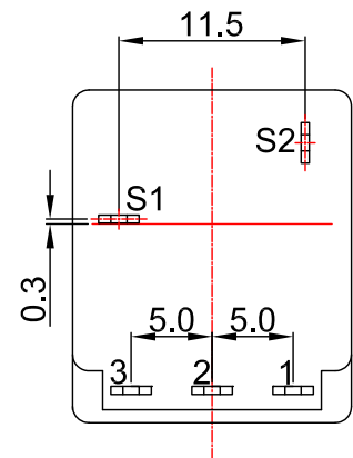
安装孔位置图 P.C.B. mounting hole detail
