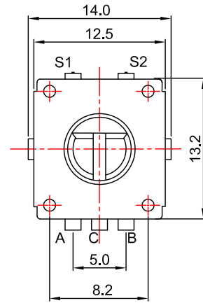
安装孔位图 P.C.B. mounting hole detail
