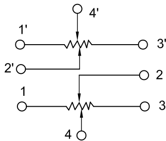
接线图 Circuit Explanation
