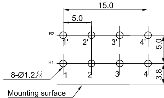
安装孔位置图 P.C.B. mounting hole detail
