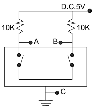
接线图 Circuit explanation
