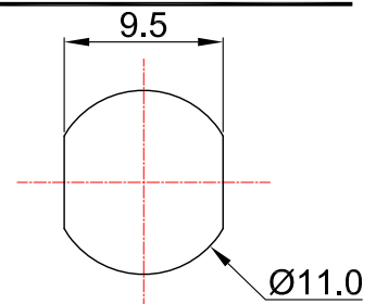
安装孔位置图 P.C.B. mounting hole detail
