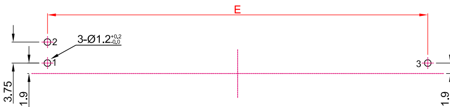
安装孔位图 P.C.B. mounting hole detail
