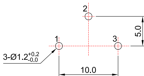
安装孔位置图 P.C.B. mounting hole detail
