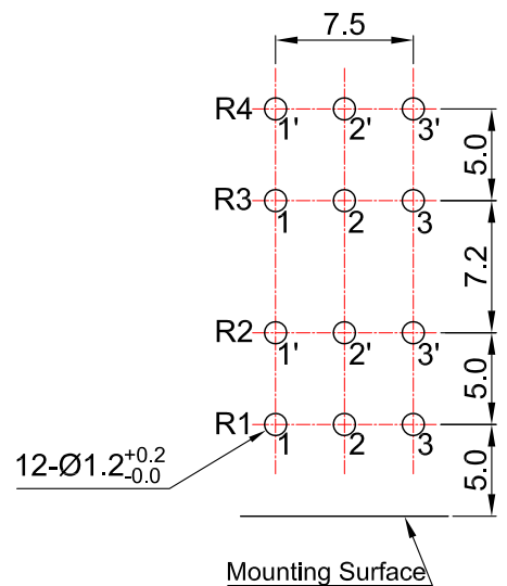
安装孔位置图 P.C.B. mounting hole detail
