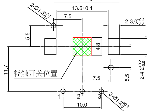
安装孔位置图 P.C.B. mounting hole detail
