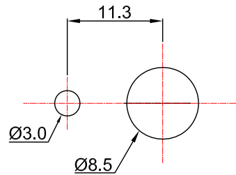
安装孔位图 P.C.B. mounting hole detail
