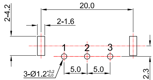
安装孔位图 P.C.B. mounting hole detail
