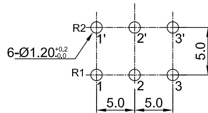
安装孔位置图 P.C.B. mounting hole detail
