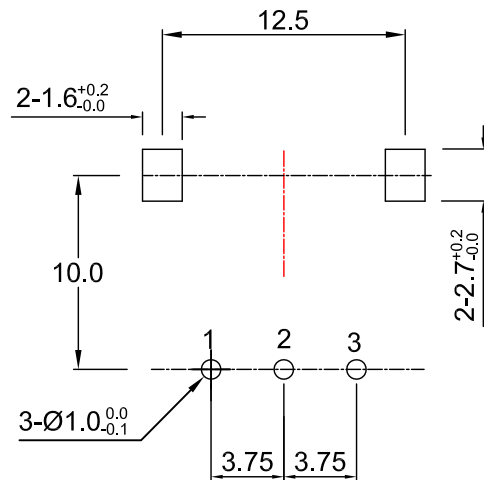
安装孔位图 P.C.B. mounting hole detail
