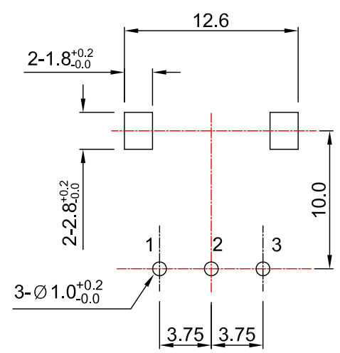
安装孔位图 P.C.B. mounting hole detail
