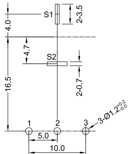
安装孔位置图 P.C.B. mounting hole detail
