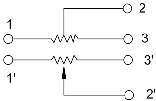
接线图 Circuit explanation
