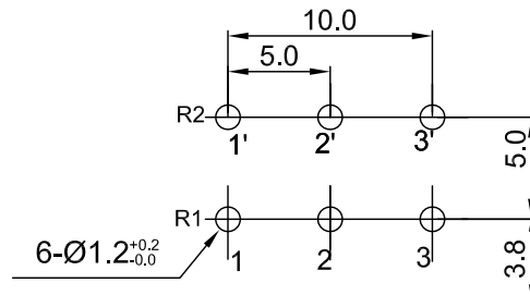
安装孔位置图 P.C.B. mounting hole detail
