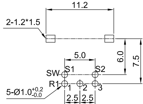
安装孔位置图 P.C.B. mounting hole detail
