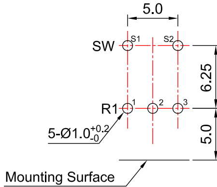
安装孔位置图 P.C.B. mounting hole detail
