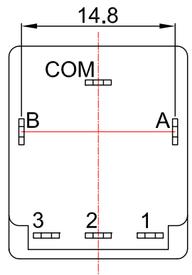
安装孔位置图 P.C.B. mounting hole detail
