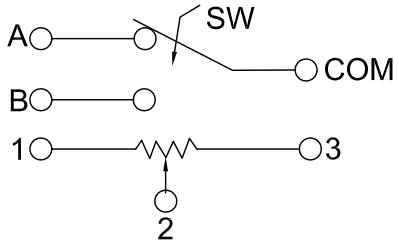
接线图 Circuit explanation
