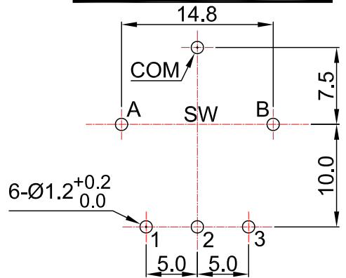
安装孔位置图 P.C.B. mounting hole detail
