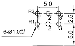
安装孔位置图 P.C.B. mounting hole detail
