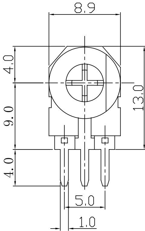
安裝孔位置圖 Mounting Hole
