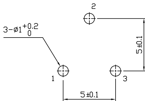
安裝孔位置圖 Mounting Hole
