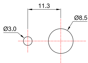
安装孔位图 Mounting hole dimensions
